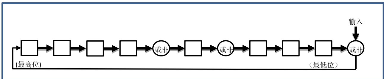
图 11.2 循环冗余校验生成器
