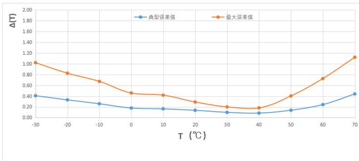
图 7- 1 MTS01B 精度误差曲线
