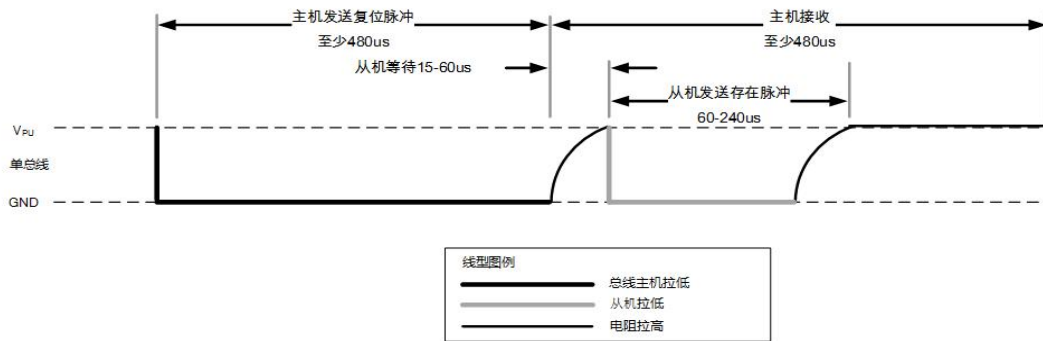
图 11.7-1 初始化时序
